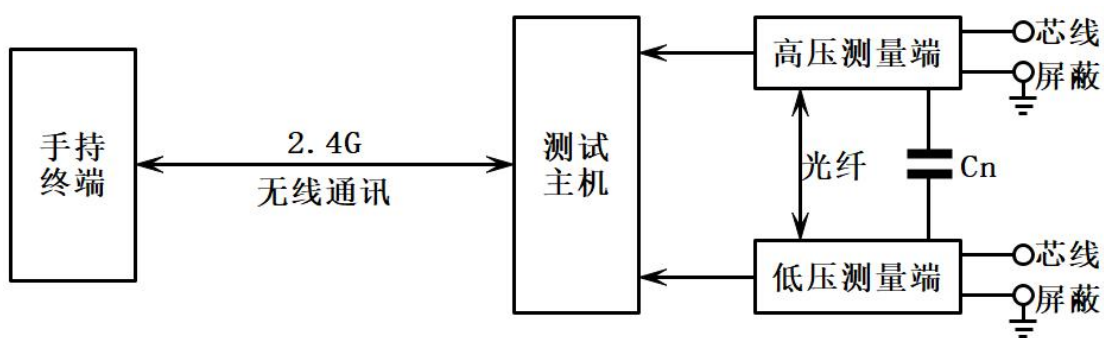
图 2—1 测量原理图
